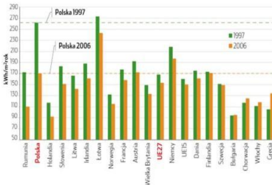
Rys. 2.1.4 Porównanie jednostkowego zużycia ciepła do ogrzewania powierzchni użytkowej budynków w wybranych krajach UE-27 w latach 1997 i 2006 [ 2.1.14]
