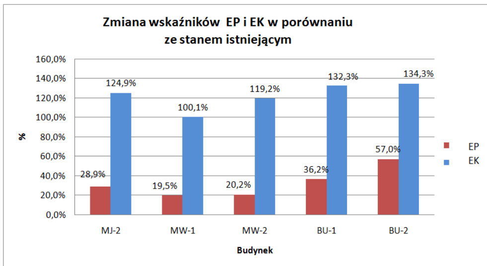
Rys. 4.2.9 Zmiana wskaźników EP i EK dla budynków w przypadku zasilania przez kocioł opalany biomasą i kolektory słoneczne
