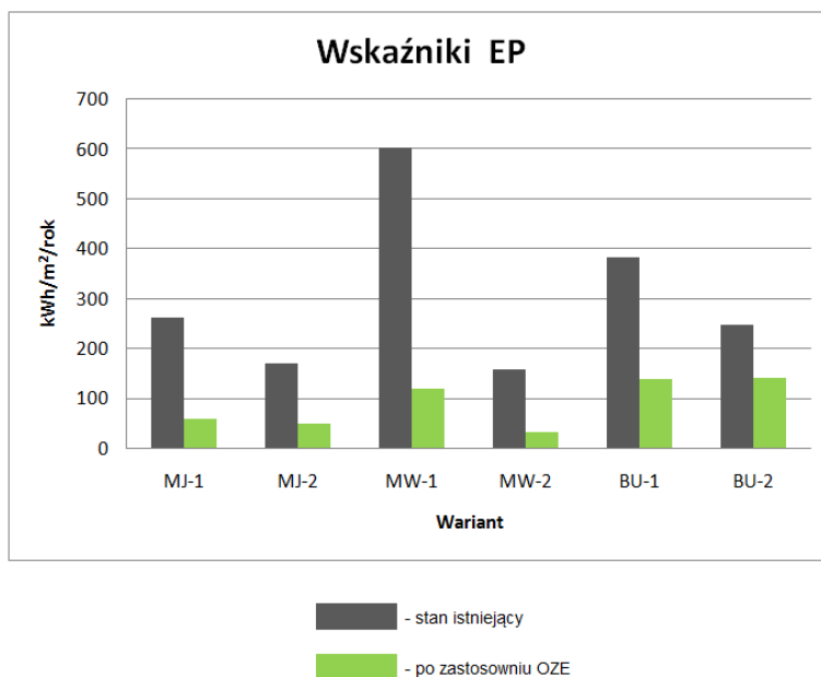
Rys. 4.2.7 Wskaźniki EP dla budynków zasilanych przez kocioł opalany biomasa i kolektory słoneczne
