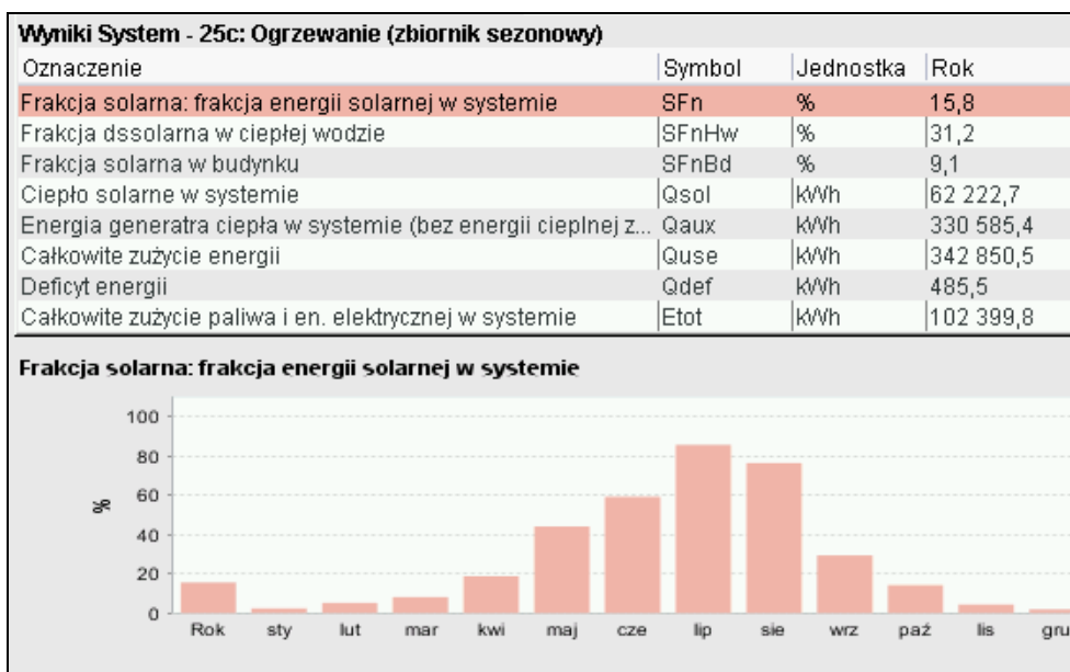
Rys. 2.2.12 Podgląd wyników dla wariantu termomodernizacji T2 przykładowego budynku użyteczności publicznej
