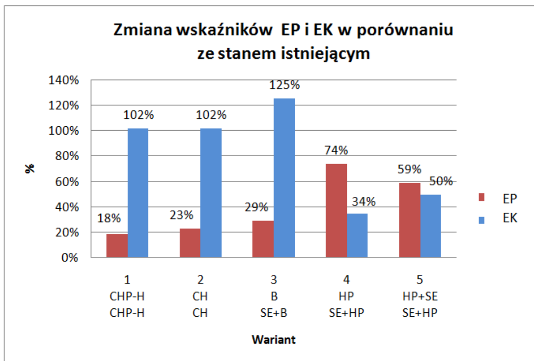
Rys. 4.1.3 Wskaźniki EP i EK dla budynku MJ-2
