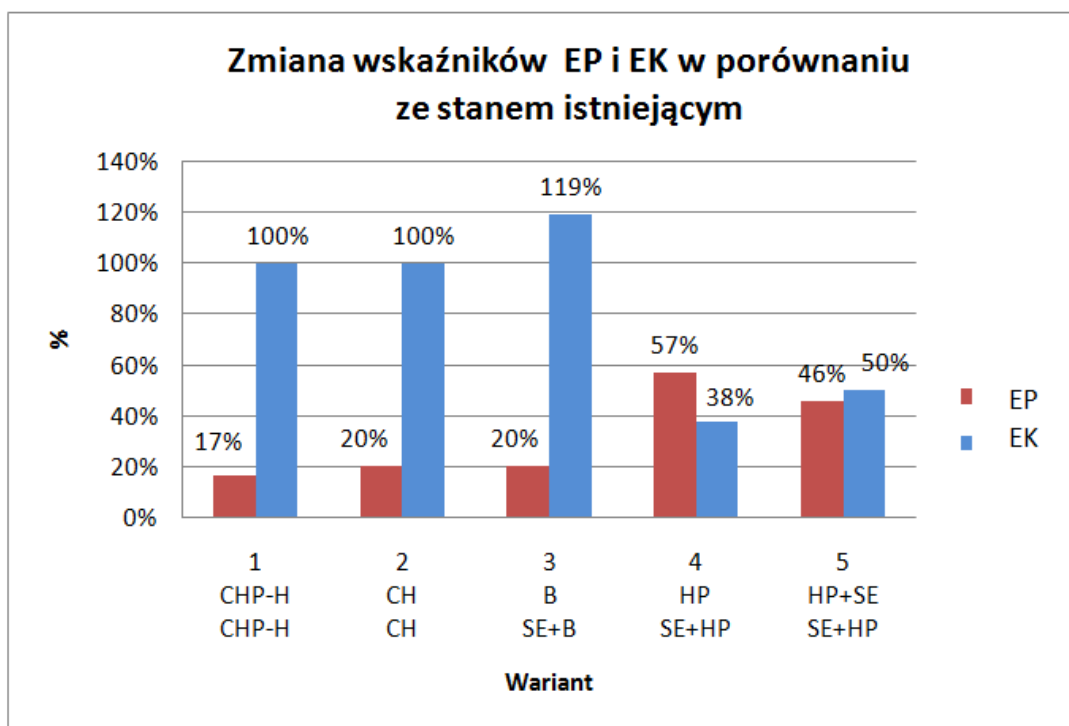
Rys. 4.1.5 Wskaźniki EP i EK dla budynku MW-2
