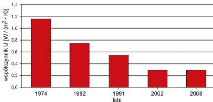
Rys. 2.1.2 Zmiany wymaganych wartości współczynnika U [W/(m 2 ·K)] dla ścian zewnętrznych budynków mieszkalnych w Polsce w latach 1974 – 2008 [2.1.9]
