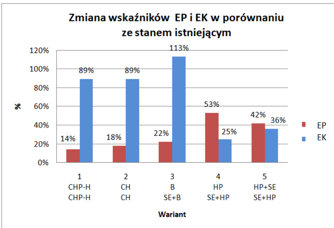
Rys. 4.1.2 Wskaźniki EP i EK dla budynku MJ-1
