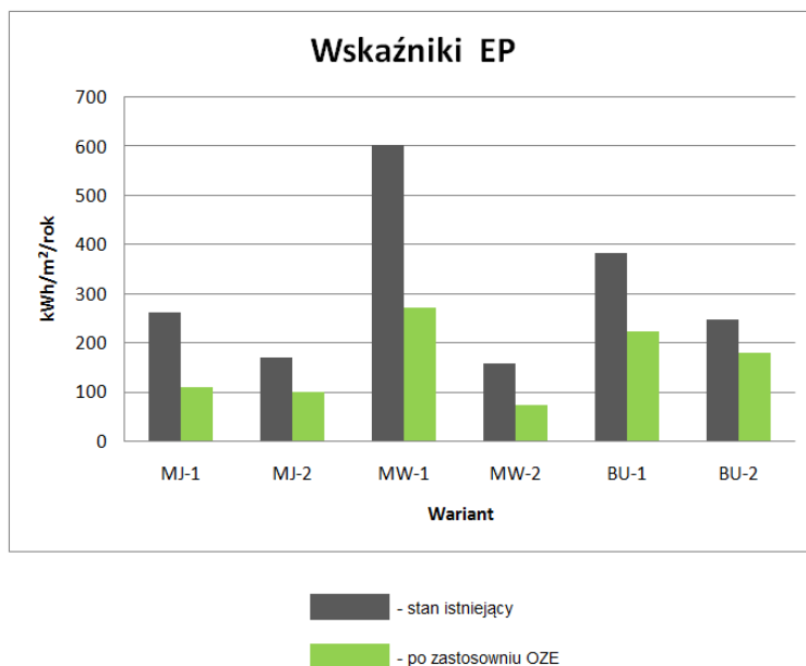
Rys. 4.2.13 Wskaźniki EP dla budynków zasilanych przez pompę ciepła i kolektory słoneczne (wspomagające system c.o.)
