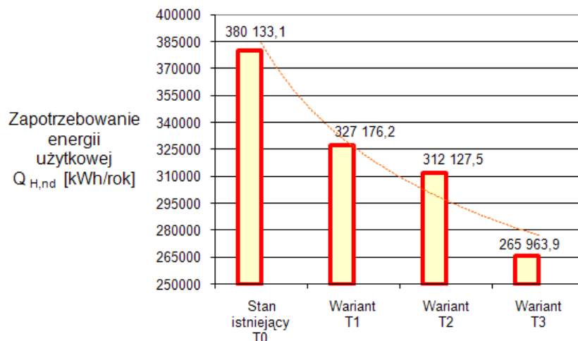
Rys. 2. 2.5 Zmiany wielkości zapotrzebowania energii użytkowej dla ogrzewania i wentylacji dla stanu istniejącego i wariantów termomodernizacji
