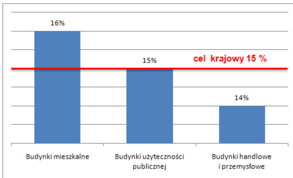
Rys. 5.6 Planowana na 2020 r. wielkość udziału energii ze źródeł odnawialnych w budynkach wobec celu krajowego (opr. własne, źródło: dane z KPD w zakresie OZE [5.19])
