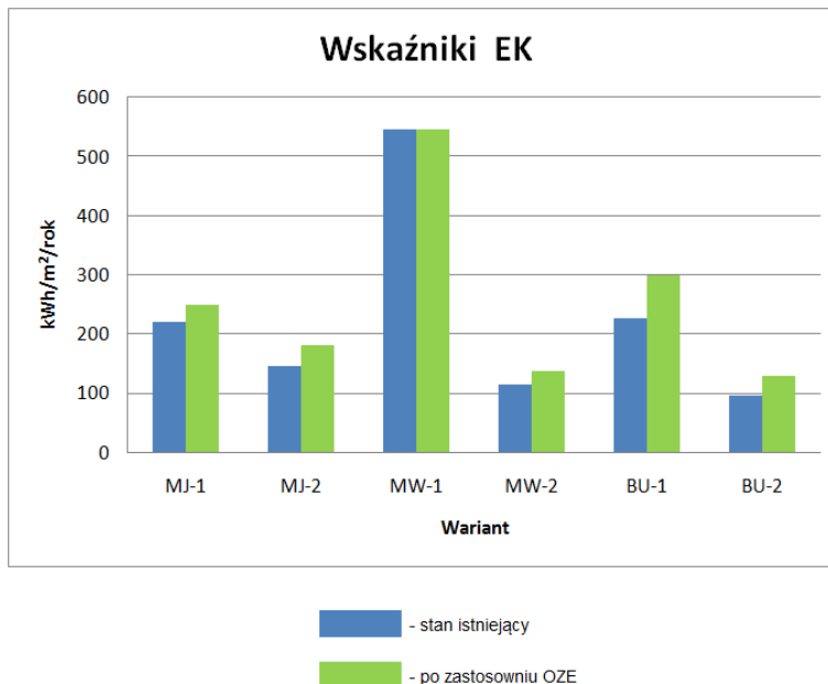
Rys. 4.2.8 Wskaźniki EK dla budynków zasilanych przez kocioł opalany biomasa i kolektory słoneczne
