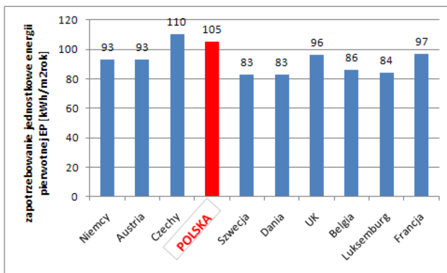
Rys. 5.3 – Wskaźnikowe zapotrzebowanie energii pierwotnej (nośnik energii – gaz ziemny) dla budynku wielorodzinnego w wybranych krajach UE ( opr. własne )
