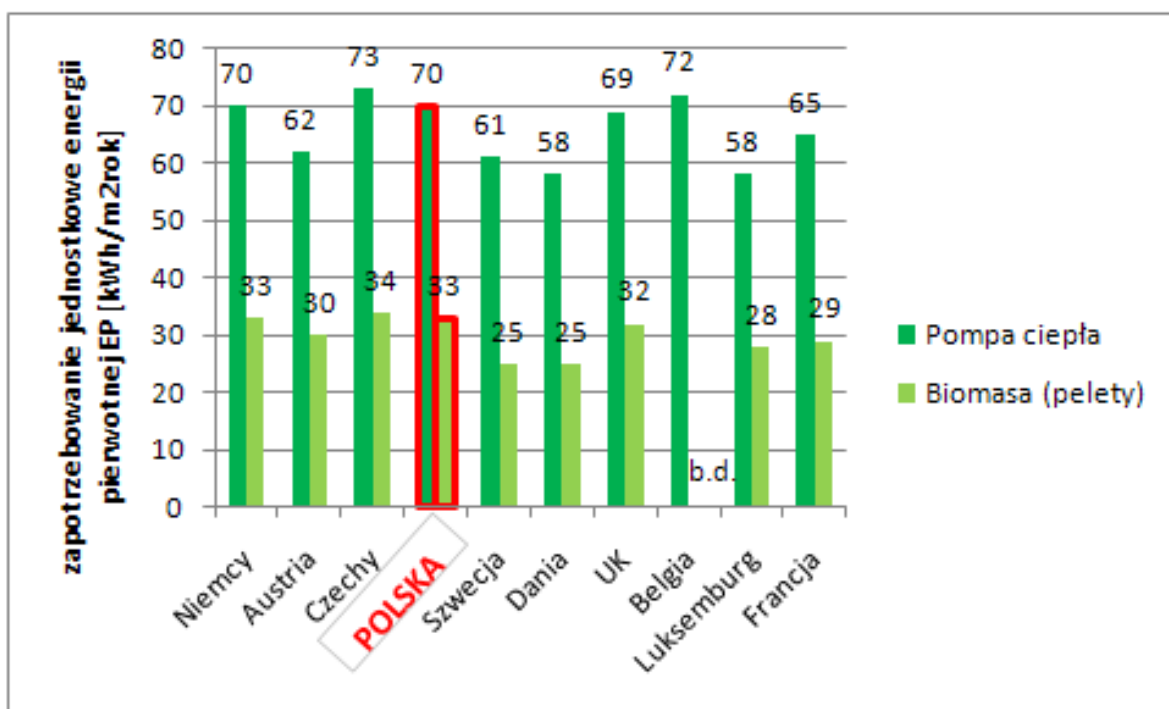
Rys. 5.4 – Wskaźnikowe zapotrzebowanie energii pierwotnej (instalacje OZE) dla budynku wielorodzinnego w wybranych krajach UE (opr. własne)
