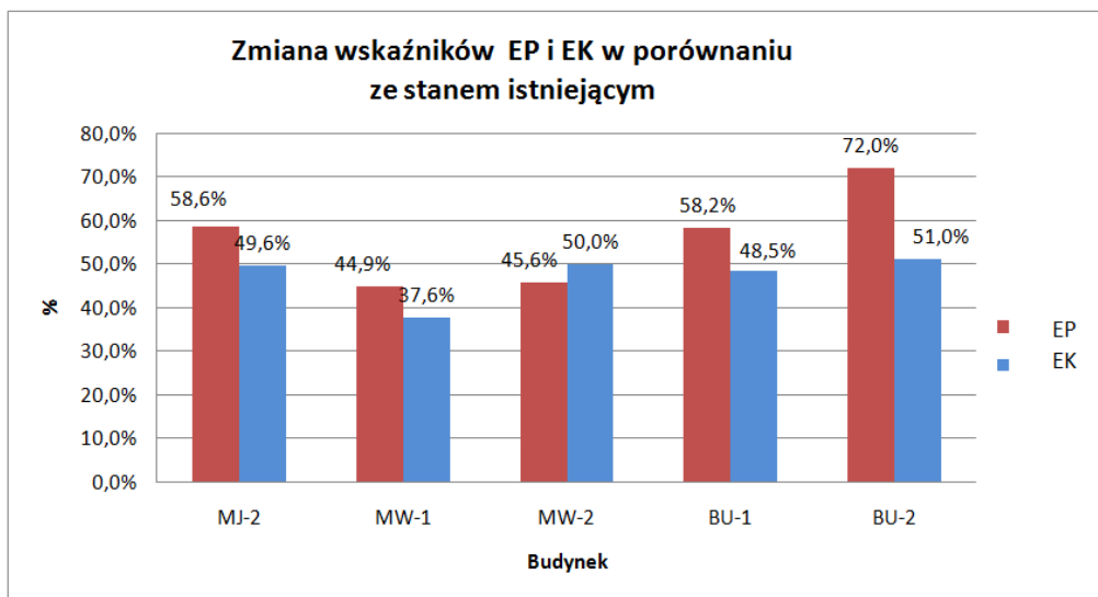
Rys. 4.2.15 Zmiana wskaźników EP i EK dla budynków w przypadku zasilania przez pompę ciepła i kolektory słoneczne (wspomagające system c.o.)
