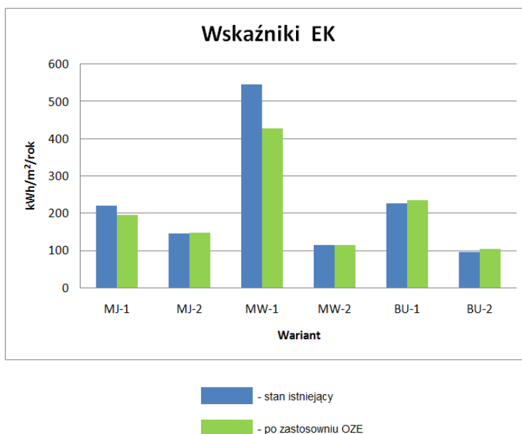
Rys. 4.2.2 - Wskaźniki EK dla budynków zasilanych z elektrociepłowni opalanej biomasa
