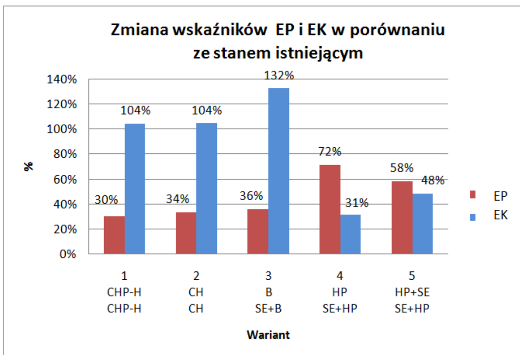
Rys. 4.1.6 Wskaźniki EP i EK dla budynku BU-1
