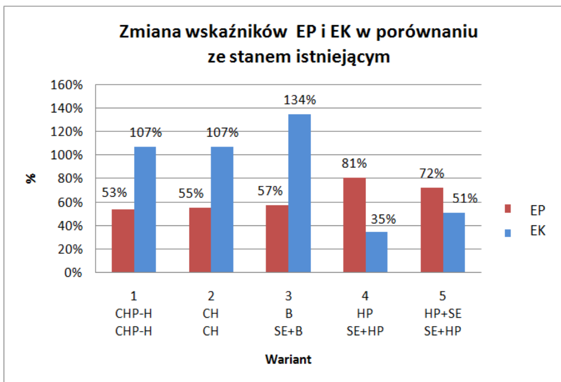
Rys. 4.1.7 Wskaźniki EP i EK dla budynku BU-2
