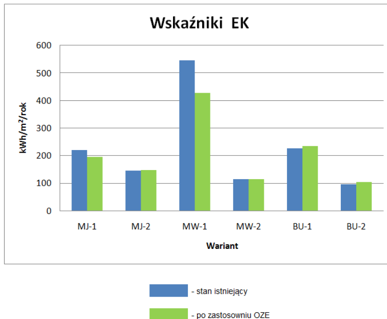
Rys. 4.2.5 Wskaźniki EK dla budynków zasilanych z ciepłowni opalanej biomasą
