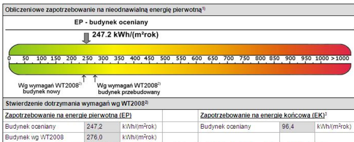
Rys. 3.4.1 Jednostkowe zapotrzebowanie na nieodnawialną energię pierwotną dla stanu istniejącego B-O
