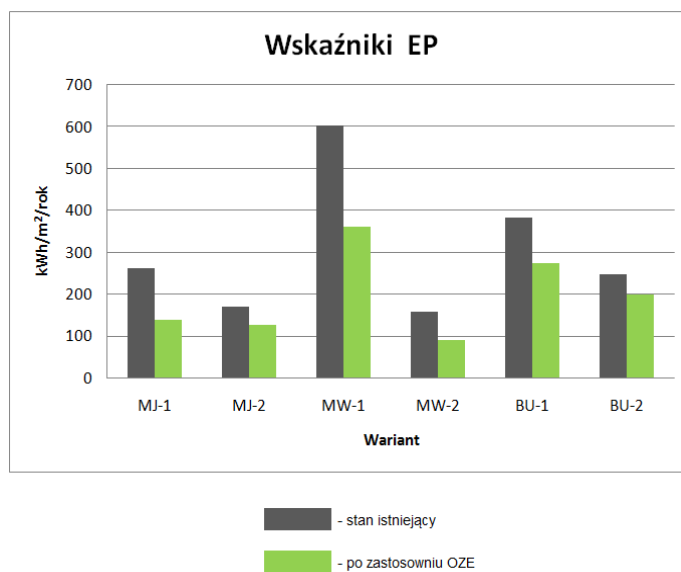
Rys. 4.2.10 Wskaźniki EP dla budynków zasilanych przez pompę ciepła i kolektory słoneczne
