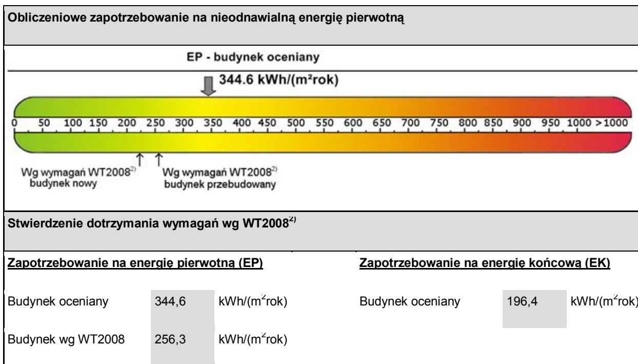
Rys. 2.2.2 Wartość wskaźników EP i EK (bez oświetlenia) ze świadectwa charakterystyki energetycznej dla wariantu T1
