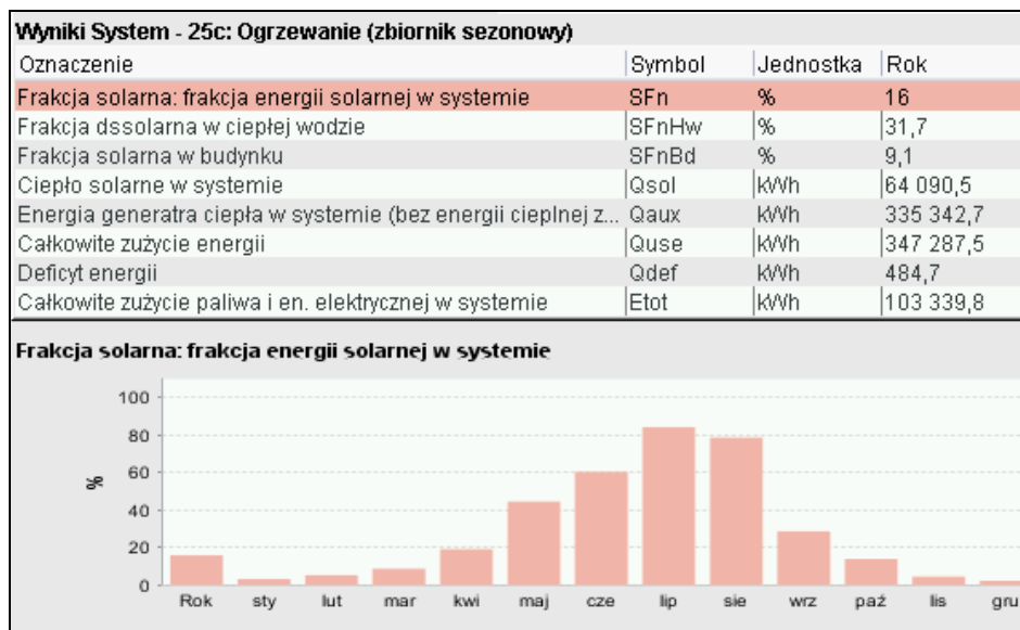
Rys. 2.2.10 Podgląd wyników dla stanu istniejącego T0 przykładowego budynku użyteczności publicznej
