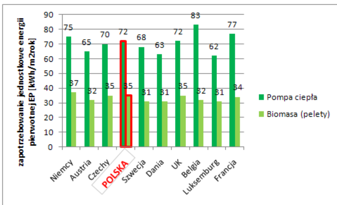
Rys. 5.4 – Wskaźnikowe zapotrzebowanie energii pierwotnej (instalacje OZE) dla budynku jednorodzinny w wybranych krajach UE ( opr. własne )
