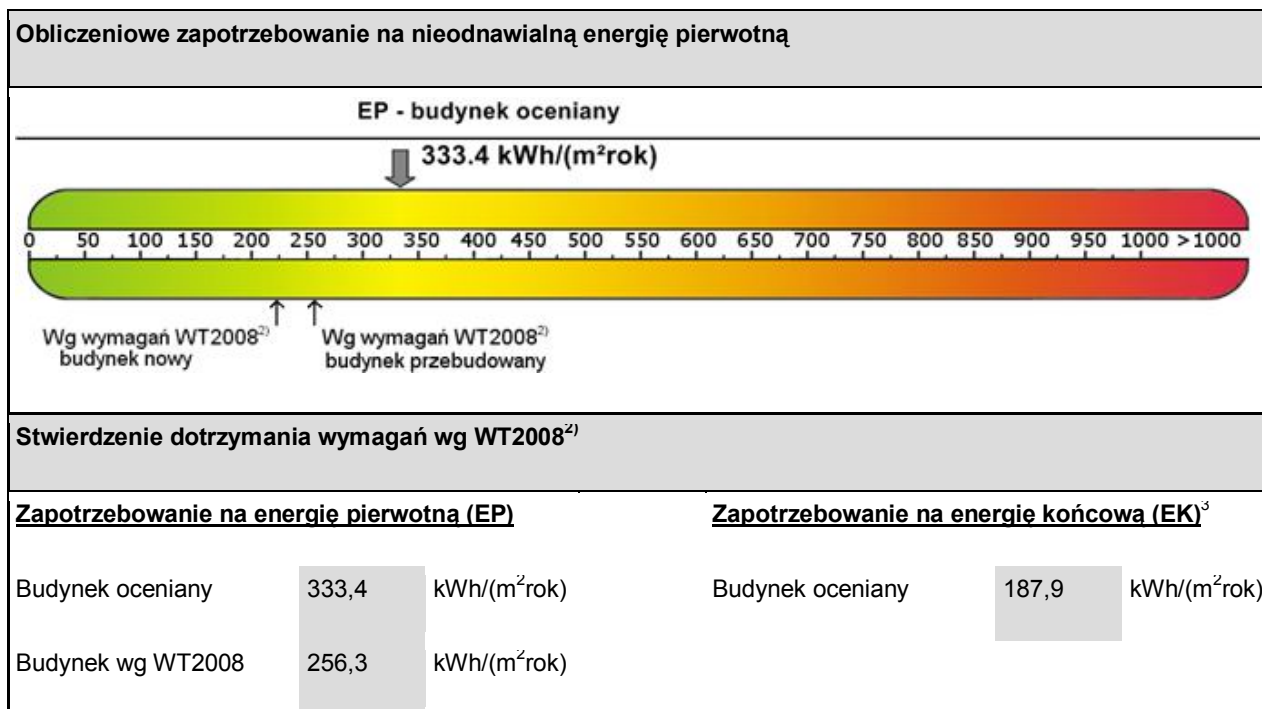
Rys. 2.2.3 Wartość wskaźników EP i EK (bez oświetlenia) ze świadectwa charakterystyki energetycznej dla wariantu T2
