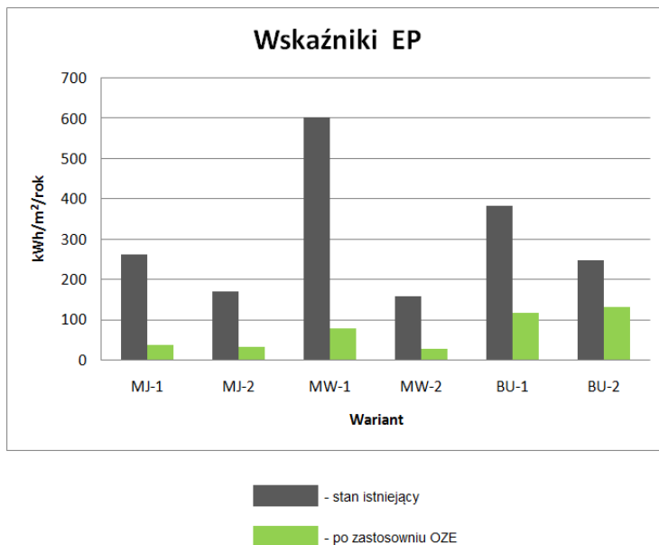
Rys. 4.2.1 Wskaźniki EP dla budynków zasilanych z elektrociepłowni opalanej biomasa
