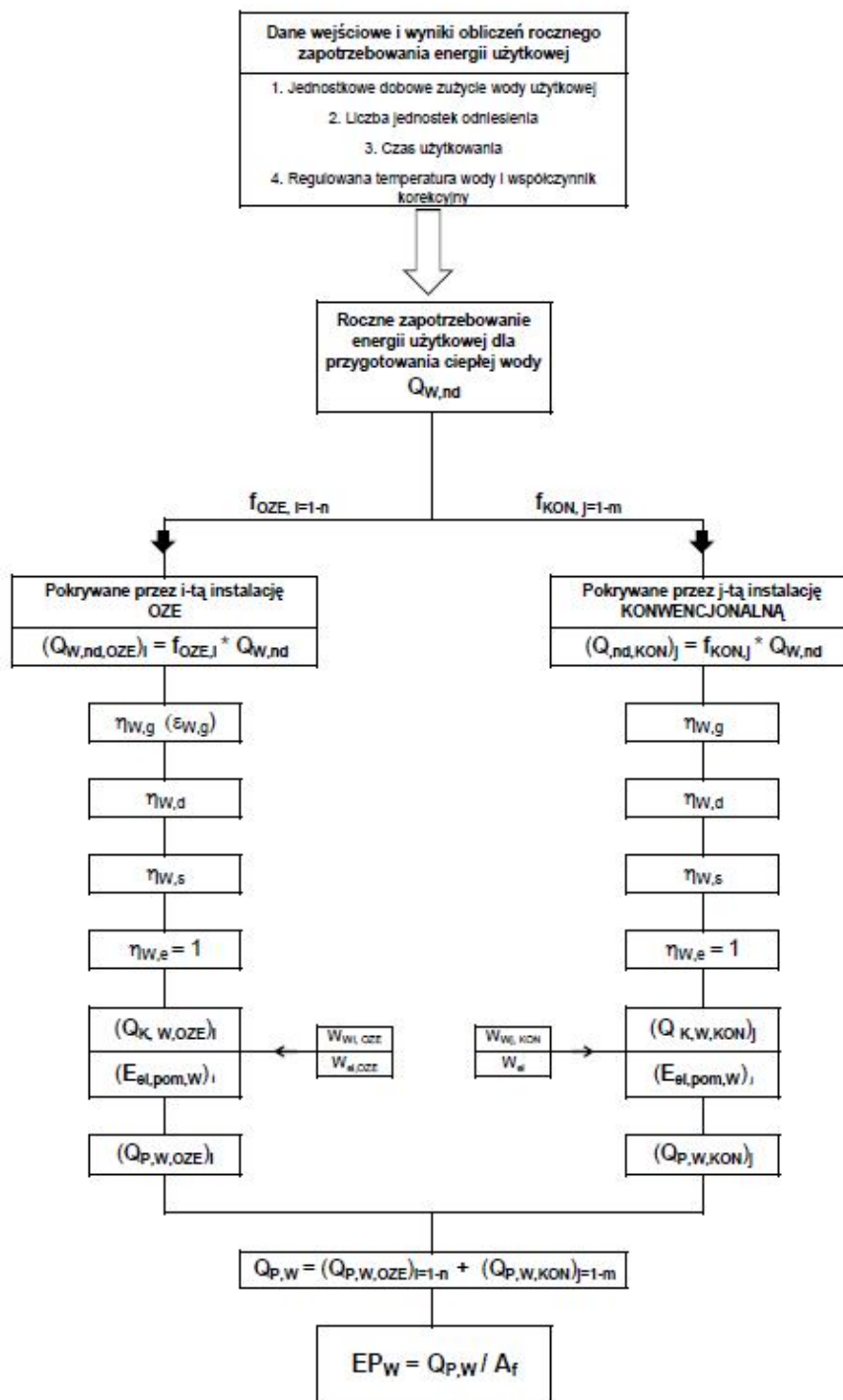
Rys. 3.3.2 Algorytm oceny poprawy charakterystyki energetycznej budynku przy stosowaniu instalacji OZE dla potrzeb przygotowania ciepłej wody użytkowej
