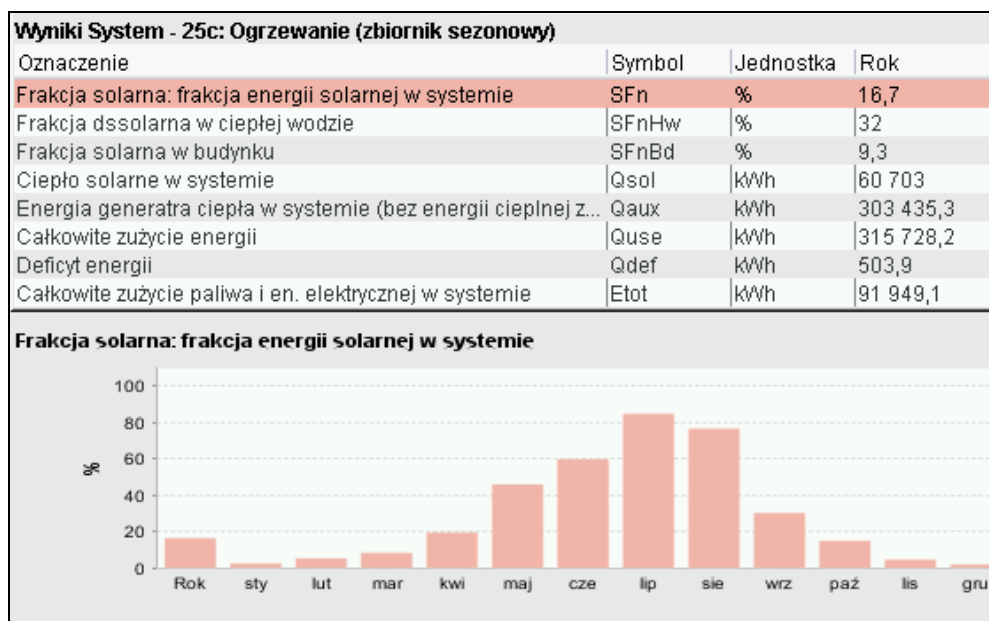
Rys. 2.2.13 Podgląd wyników dla wariantu termomodernizacji T3 przykładowego budynku użyteczności publicznej
