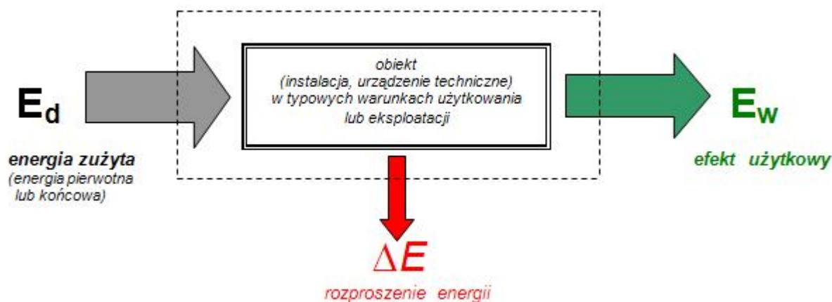
Rys. 5.1 – Bilans energii dla określenia efektywności energetycznej obiektu ( opr. własne )
