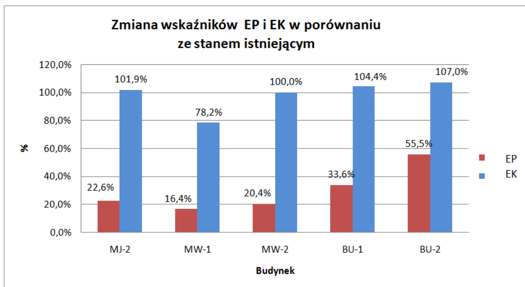
Rys. 4.2.6 Zmiana wskaźników EP i EK dla budynków w przypadku zasilania w ciepło z ciepłowni opalanej biomasą
