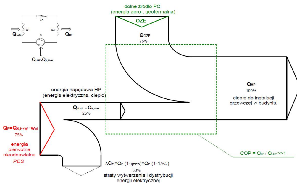
Rys. 3.2.3 Efektywność wykorzystania energii pierwotnej nieodnawialnej i zasobów OZE w pompie ciepła (opracowanie własne)
