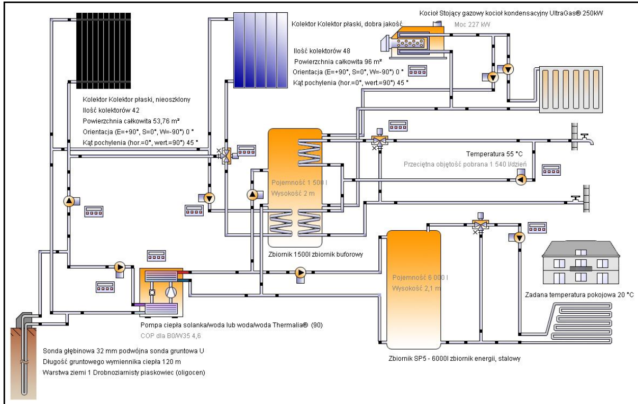
Rys. 2.2.9 Schemat doboru urządzeń przy zastosowaniu instalacji z OZE dla stanu istniejącego – wariant T0 (szablon programu POLYSUN)
