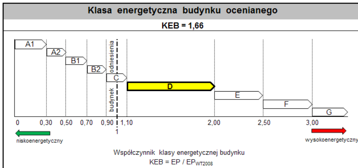
Rys. 2.4.1 Propozycja wprowadzenia klasy energetycznej w świadectwie charakterystyki energetycznej budynku (opracowanie własne)
