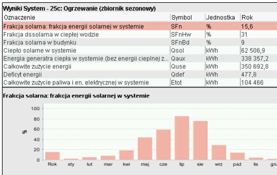
Rys. 2.2.11 Podgląd wyników dla wariantu termomodernizacji T1 przykładowego budynku użyteczności publicznej
