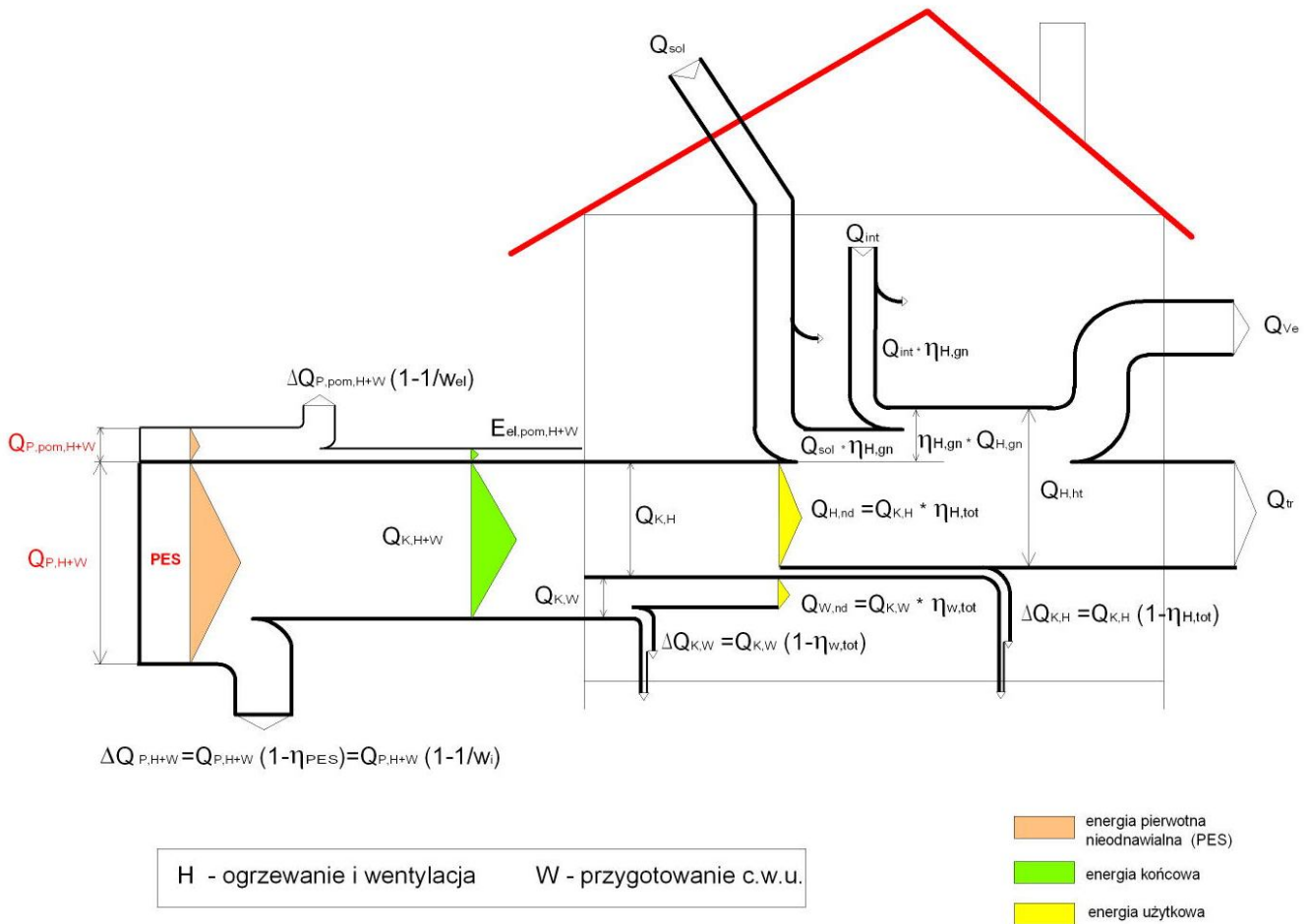
Rys. 2.1.1 Efektywność wykorzystania w budynku nieodnawialnej energii pierwotnej (opracowanie własne)
