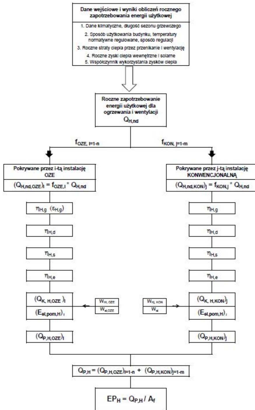
Rys. 3.3.1 Algorytm oceny poprawy charakterystyki energetycznej budynku przy stosowaniu instalacji OZE dla potrzeb ogrzewania i wentylacji
