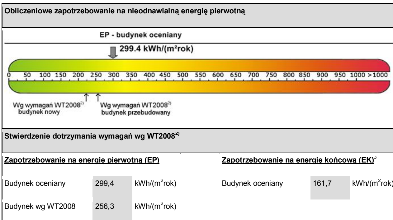
Rys. 2.2.4 Wartość wskaźników EP i EK (bez oświetlenia) ze świadectwa charakterystyki energetycznej dla wariantu T3
