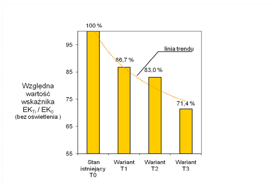
Rys. 2.2.7 Zmiany względnej wielkości wskaźnika jednostkowego zapotrzebowania energii końcowej EK dla ogrzewania i wentylacji (dla wariantów termomodernizacji w stosunku do stanu istniejącego)
