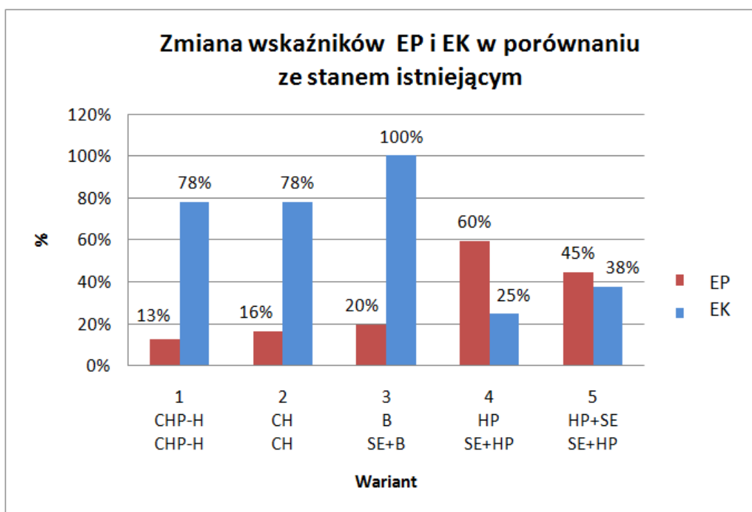
Rys. 4.1.4 Wskaźniki EP i EK dla budynku MW-1
