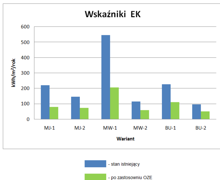
Rys. 4.2.14 Wskaźniki EK dla budynków zasilanych przez pompę ciepła i kolektory słoneczne (wspomagające system c.o.)
