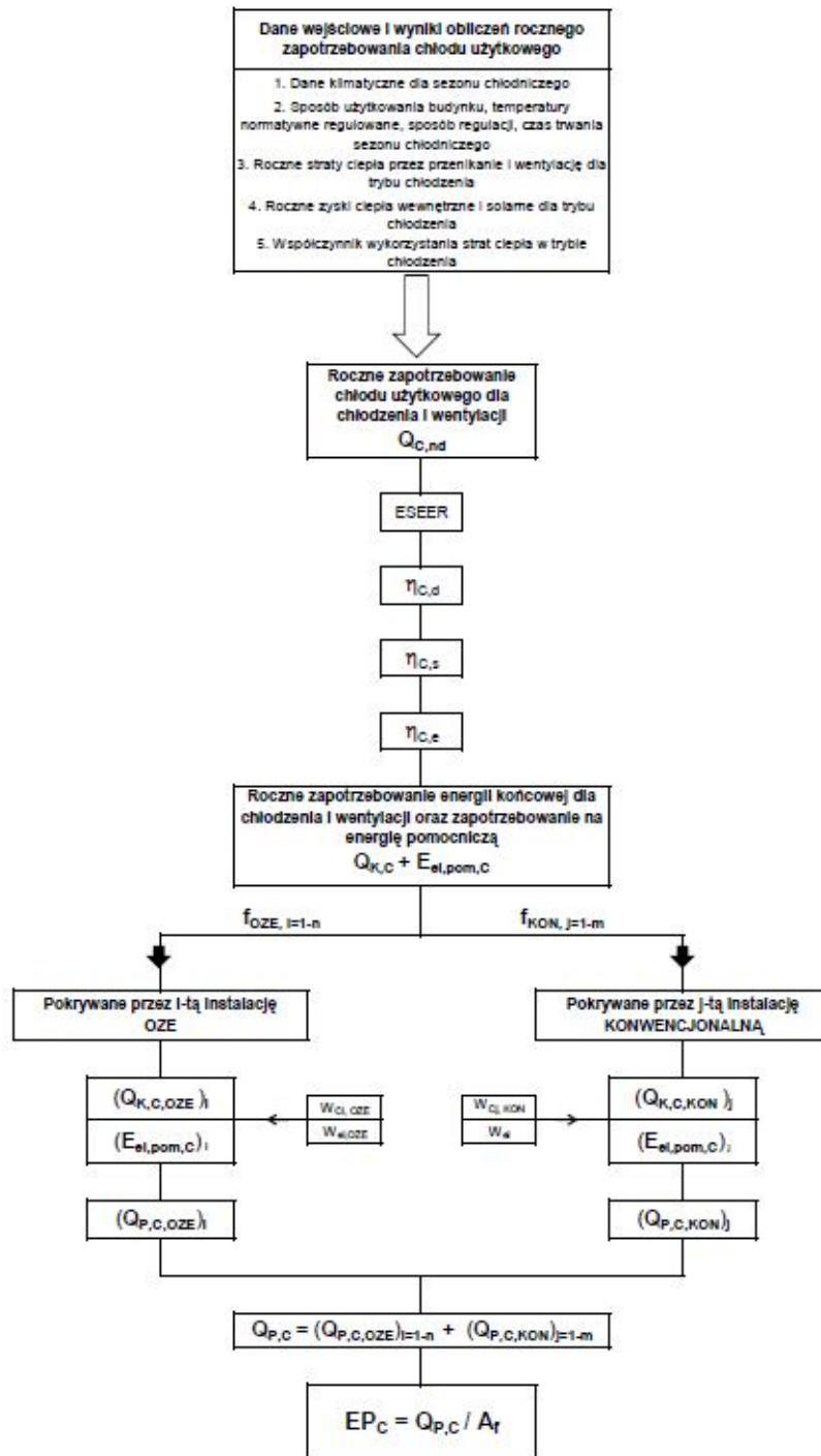
Rys. 3.3.3 Algorytm oceny poprawy charakterystyki energetycznej budynku przy stosowaniu instalacji OZE dla potrzeb chłodzenia i wentylacji
