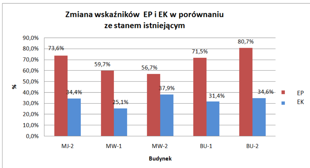
Rys. 4.2.12 Zmiana wskaźników EP i EK dla budynków w przypadku zasilania przez pompę ciepła i kolektory słoneczne
