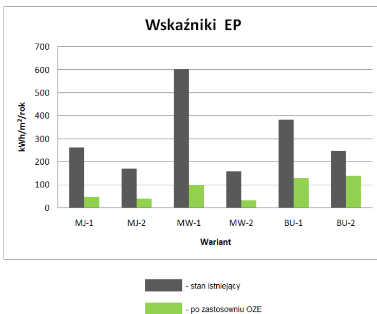
Rys. 4.2.4 Wskaźniki EP dla budynków zasilanych z ciepłowni opalanej biomasą
