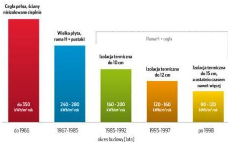
Rys. nr 2.1.3 Wskaźniki zużycia energii [kWh/m 2 ·rok] do ogrzewania budynków w Polsce na przestrzeni lat [2.1.14]
