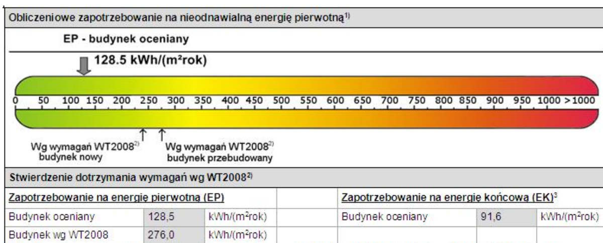
Rys. 3.4.5 Jednostkowe zapotrzebowanie na nieodnawialną energię pierwotną dla wariantu B-OZE4
