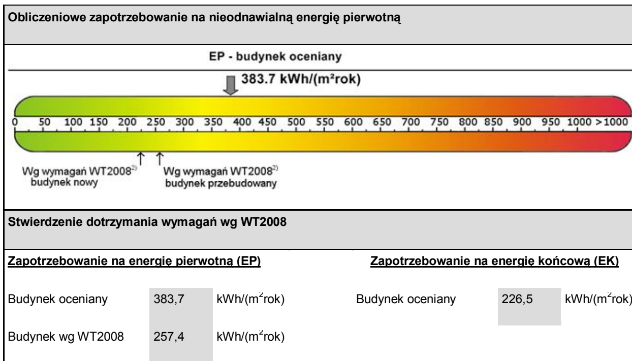
Rys. 2.2.1 Wartość wskaźników EP i EK (bez oświetlenia) ze świadectwa charakterystyki energetycznej dla stanu istniejącego T0
