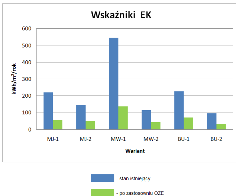
Rys. 4.2.11 Wskaźniki EK dla budynków zasilanych przez pompę ciepła i kolektory słoneczne
