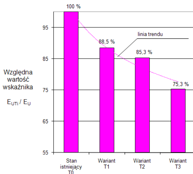
Rys. 2.2.6 Zmiany względnej wielkości wskaźnika jednostkowego zapotrzebowania energii użytkowej EU dla ogrzewania i wentylacji (dla wariantów termomodernizacji w stosunku do stanu istniejącego)
