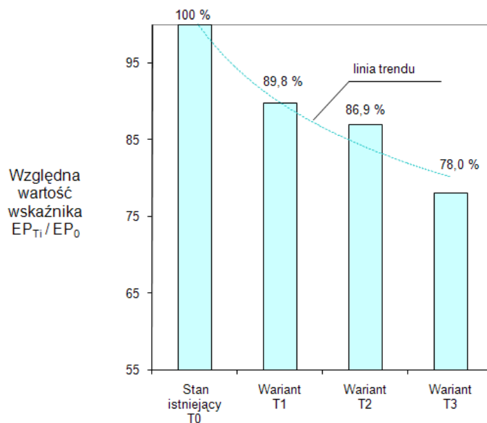
Rys. 2.2.8 Zmiany względnej wielkości wskaźnika jednostkowego zapotrzebowania nieodnawialnej energii pierwotnej EP dla ogrzewania i wentylacji (dla wariantów termomodernizacji w stosunku do stanu istniejącego)
