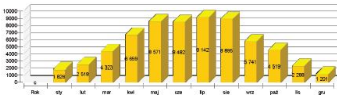
Ciepło solarne w systemie [Q sol ]
