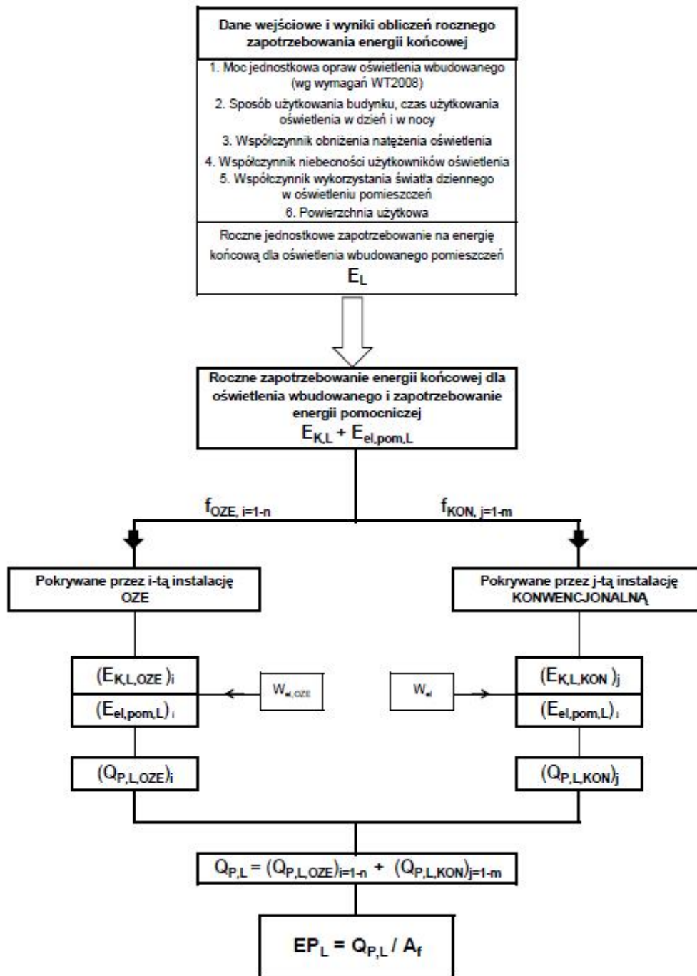
Rys. 3.3.4 Algorytm oceny poprawy charakterystyki energetycznej budynku przy stosowaniu instalacji OZE dla potrzeb oświetlenia wbudowanego
