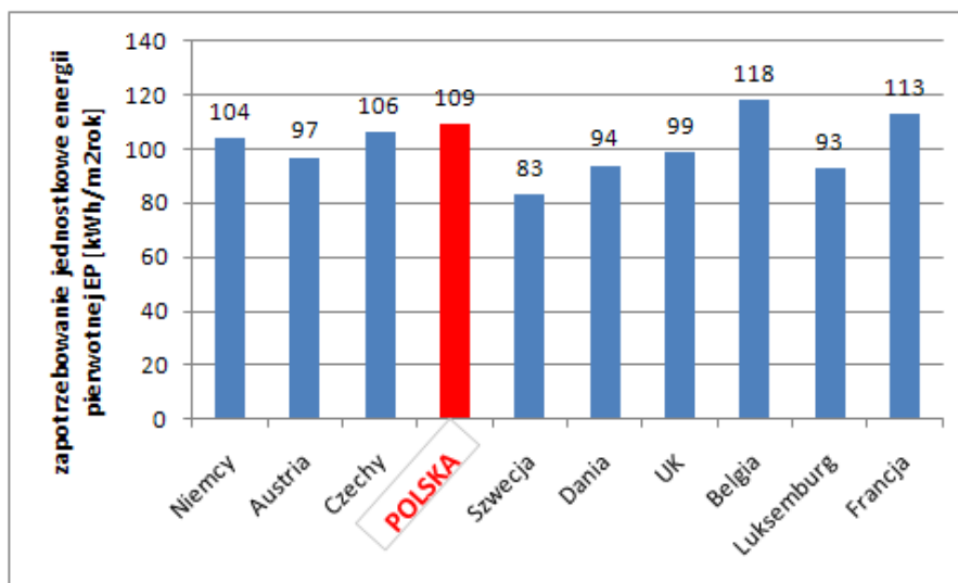
Rys. 5.2 – Wskaźnikowe zapotrzebowanie energii pierwotnej (nośnik energii – gaz ziemny) dla budynku jednorodzinnego w wybranych krajach UE ( opr. własne )
