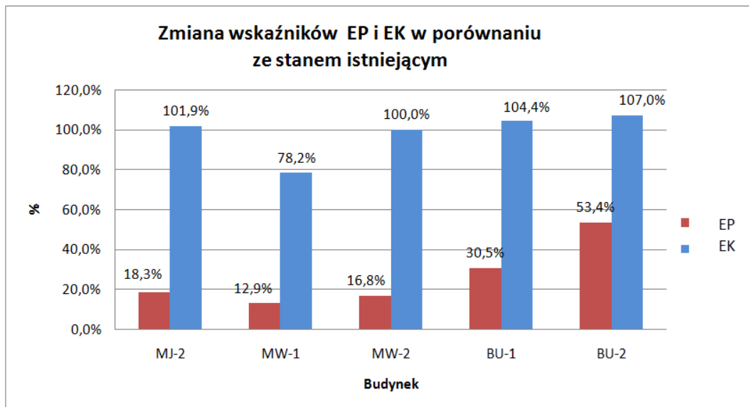
Rys. 4.2.3 Zmiana wskaźników EP i EK dla budynków w przypadku zasilania w ciepło z elektrociepłowni opalanej biomasą
