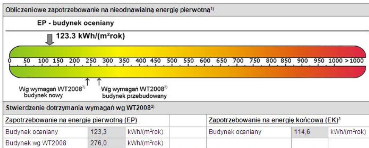
Rys. 3.4.2 Jednostkowe zapotrzebowanie na nieodnawialną energię pierwotną dla wariantu B-OZE1
